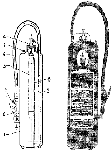
Πυροσβεστήρες ξηράς σκόνης με εσωτερικό φιαλίδιο
